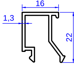
Profil No: 3899 Gramaj : 0,230 kg/m
