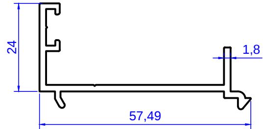
Profil No: 3824 Gramaj : 0,516 kg/m
