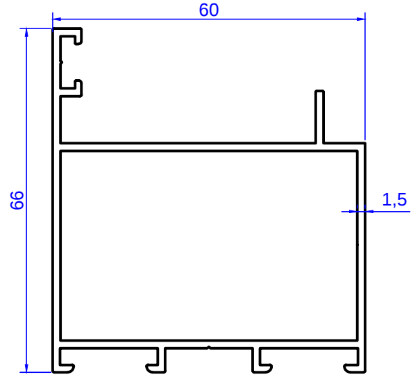
Profil No: 1961 Gramaj : 1,059
