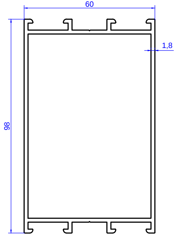
Profil No: 2553 Gramaj : 1,678 kg/m
