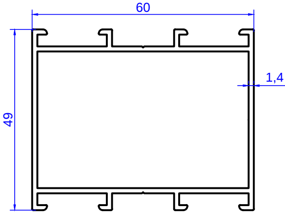
Profil No: 1960 Gramaj : 0.942 kg/m
