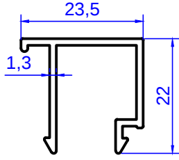
Profil No: 3823 Gramaj : 0,252 kg/m
