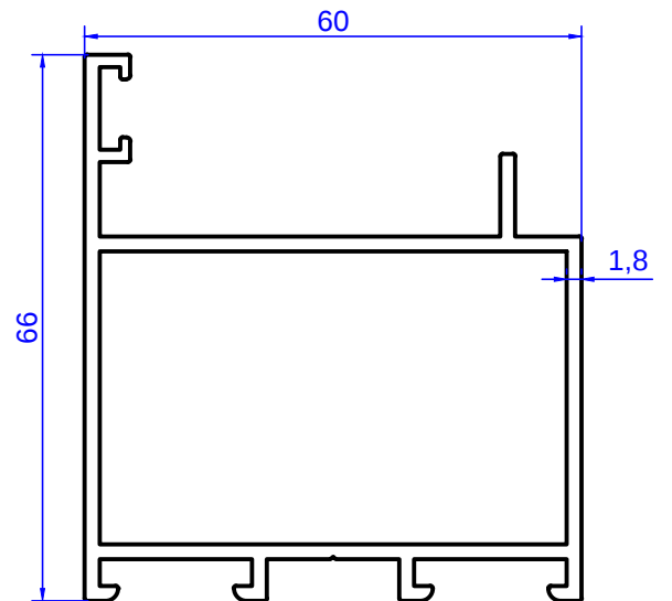
Profil No: 3822 Gramaj : 1,315 kg/m
