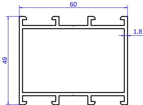
Profil No: 3821 Gramaj : 1,200 kg/m
