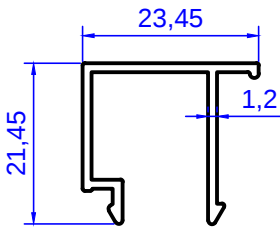
Profil No: 1964 Gramaj : 0.229 kg/m
