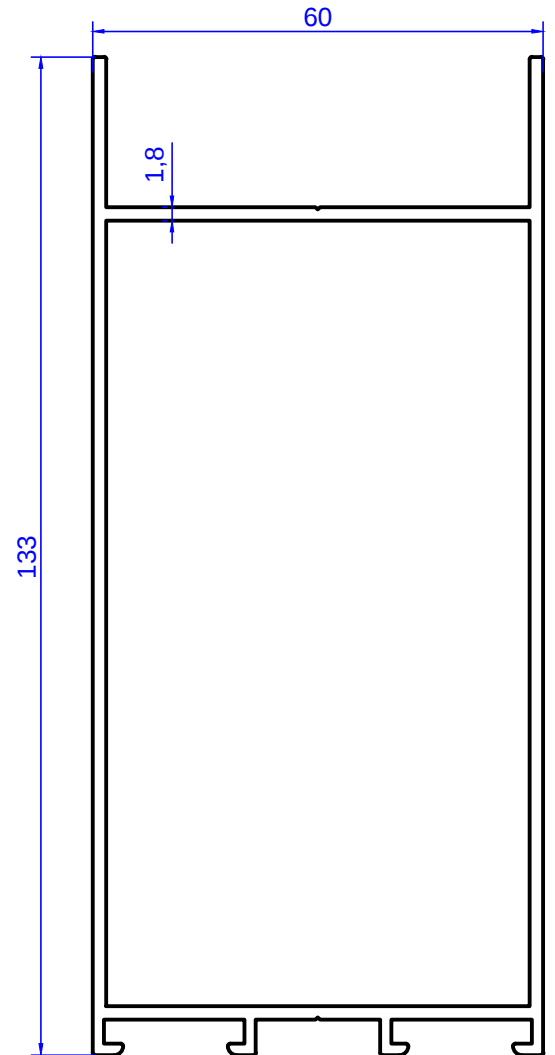
Profil No: 1962 Gramaj : 1,912 kg/m
