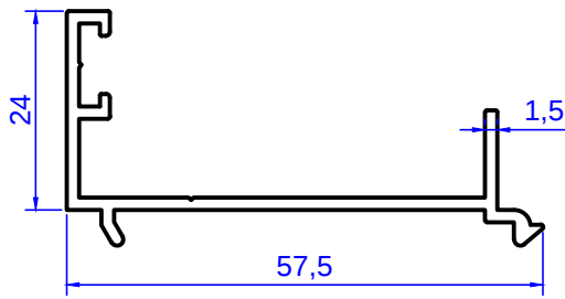
Profil No: 1963 Gramaj : 0.442 kg/m
