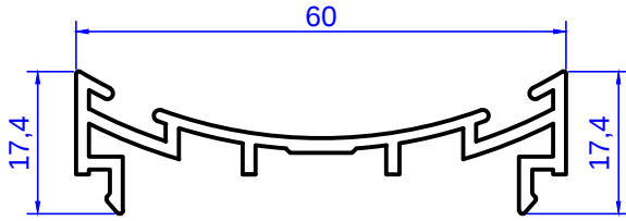
Profil No: 2571 Gramaj : 0,530 kg/m
