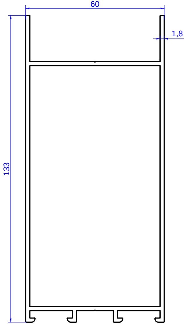
Profil No: 3820 Gramaj : 1,933 kg/m
