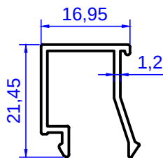
Profil No: 1965 Gramaj : 0.208 kg/m
