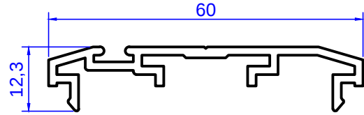
Profil No: 2570 Gramaj : 0,499 kg/m
